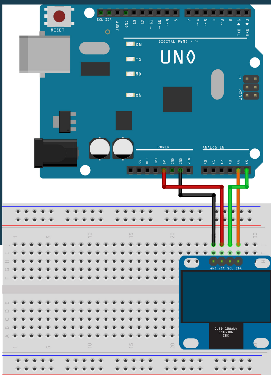
Figura 3 – Conexão dos pinos SCL e SDA do display OLED às portas A5 e A4 do Arduino
