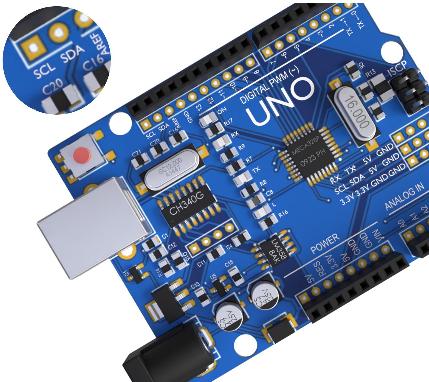
Figura 4 – Detalhe das portas SCL e SDA em versão do Arduino Uno R3
