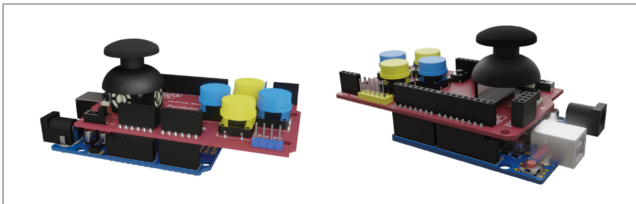
Figura 8 - Acoplando o joystick shield à placa Arduino
