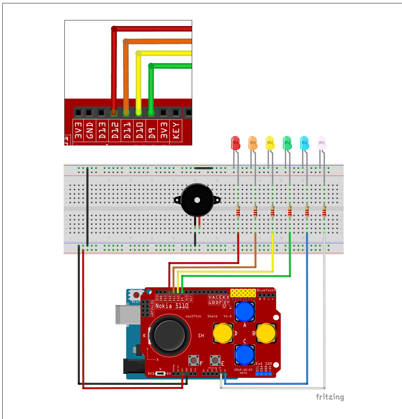
Figura 14 - Conexão dos LEDs às portas digitais do joystick shield
