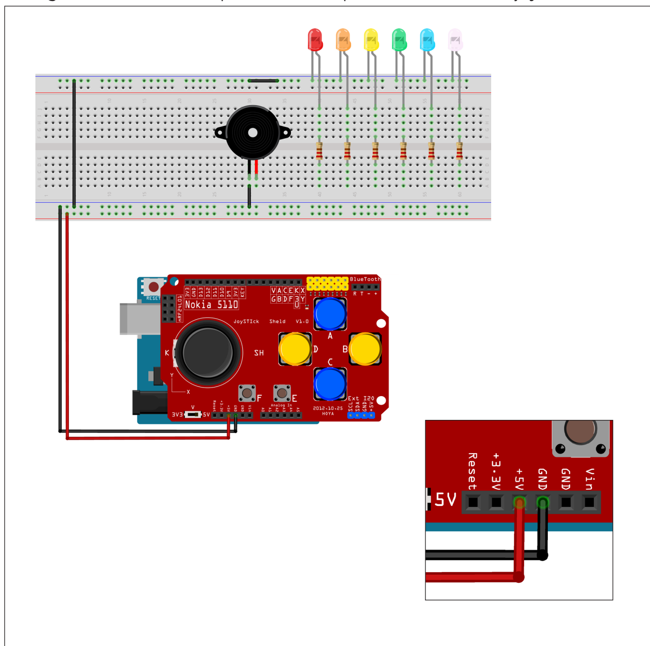
Figura 12 - Conexão da protoboard às portas 5 V e GND do joystick shield
