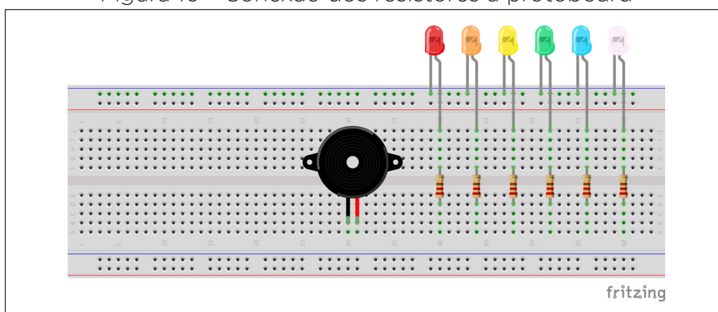
Figura 10 - Conexão dos resistores à protoboard
