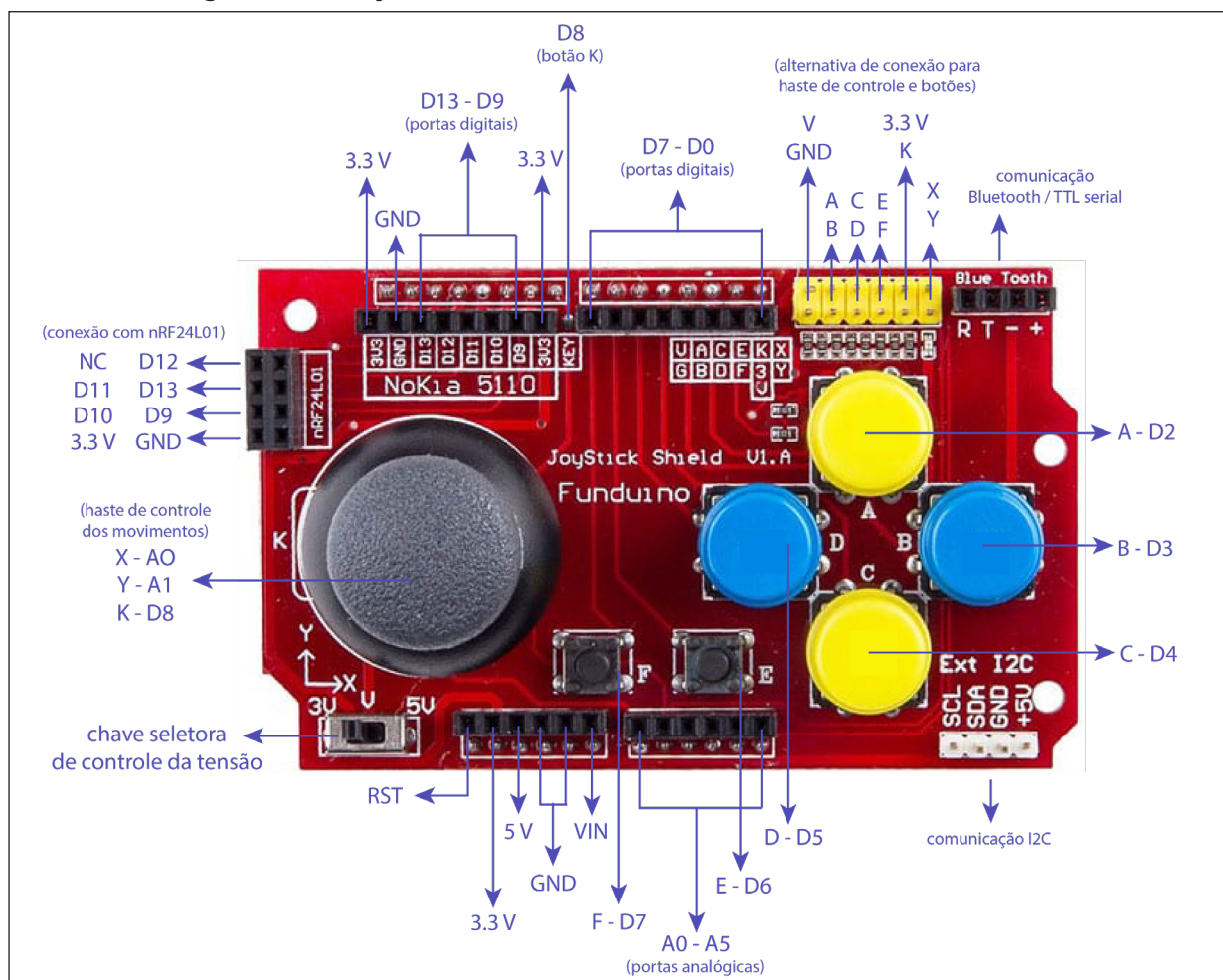
Figura 4 - Joystick shield e suas conexões com o Arduino
