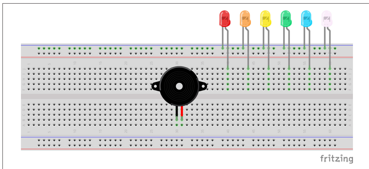
Figura 9 - Conexão de buzzer e LEDs à protoboard
